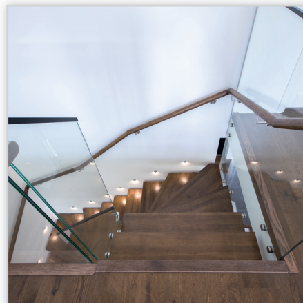
Schody jednobelkowe z balustradą float i pochwytym drewnianym.
